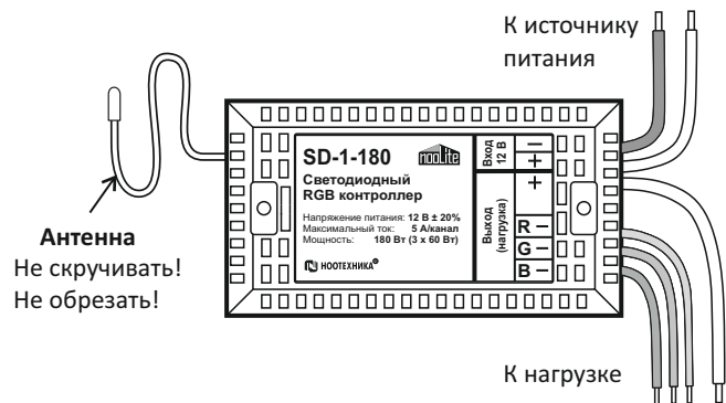
Вид спереди блока SD-1-180
