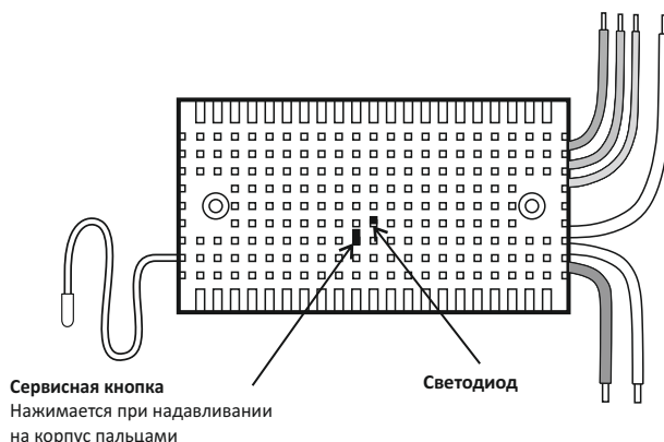
Вид сзади блока SD-1-180
